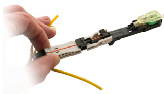
Mechanický konektor
